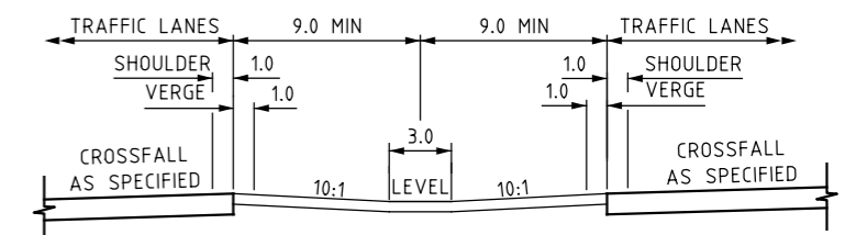
SECTION A-A
